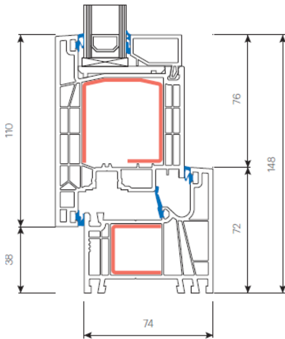
Drzwi przejściowe – otwieranie zewn. (7001+7084)
