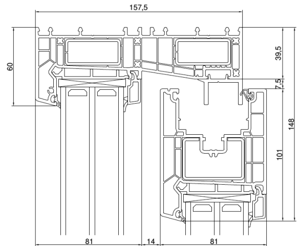
KOMPLETTE KONSTRUKTION – VERTIKALE ANSICHT
