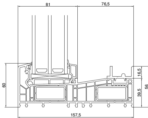
FIX – VERTIKALE ANSICHT
