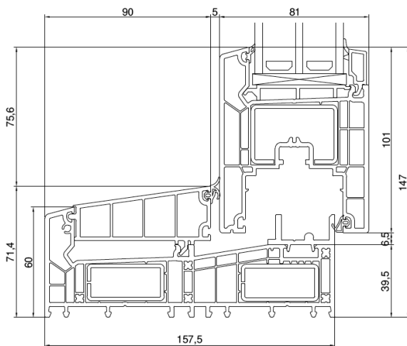
MOBILE TÜR – VERTIKALE ANSICHT
