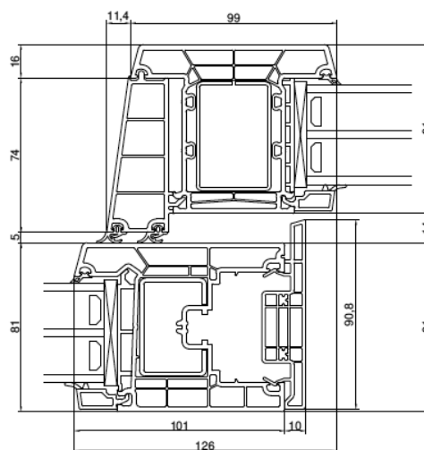
KOMPLETTE KONSTRUKTION – HORIZONTALANSICHT
