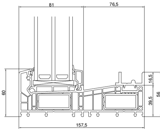
PARTIE FIXE – COUPE VERTICALE
