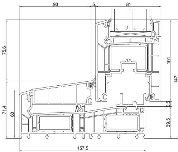
PARTIE MOBILE – COUPE VERTICALE
