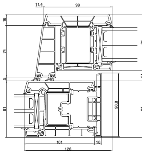
CONSTRUCTION COMPLÈTE – COUPE HORIZONTALE
