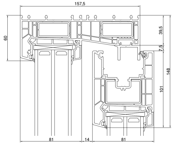
CONSTRUCTION COMPLÈTE – COUPE VERTICALE
