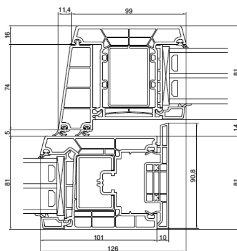
CONSTRUZIONE COMPLETA – VISTA ORIZZONTALE
